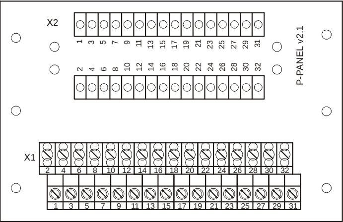
Рисунок 2. Схема расположения элементов.
