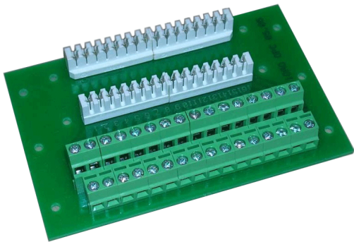
Рисунок 1. Внешний вид патч-панели.
